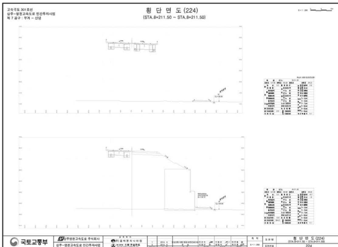
【그림 78.5】 단면도
