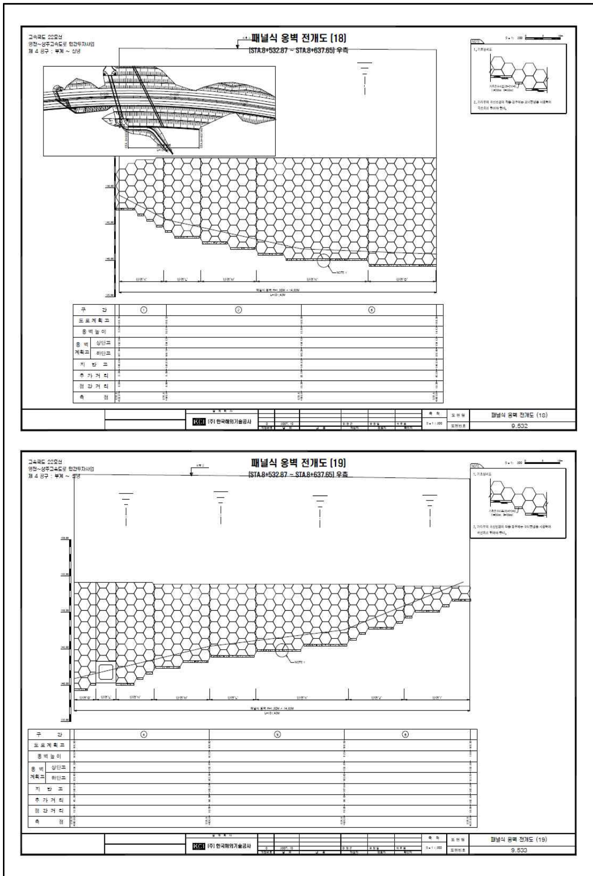
【그림 12.4】 전개도(계속)
