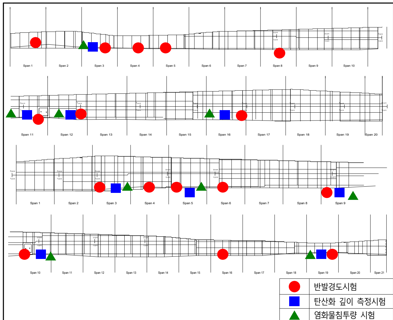
【그림 78.6】 콘크리트 재료시험 조사 위치도
