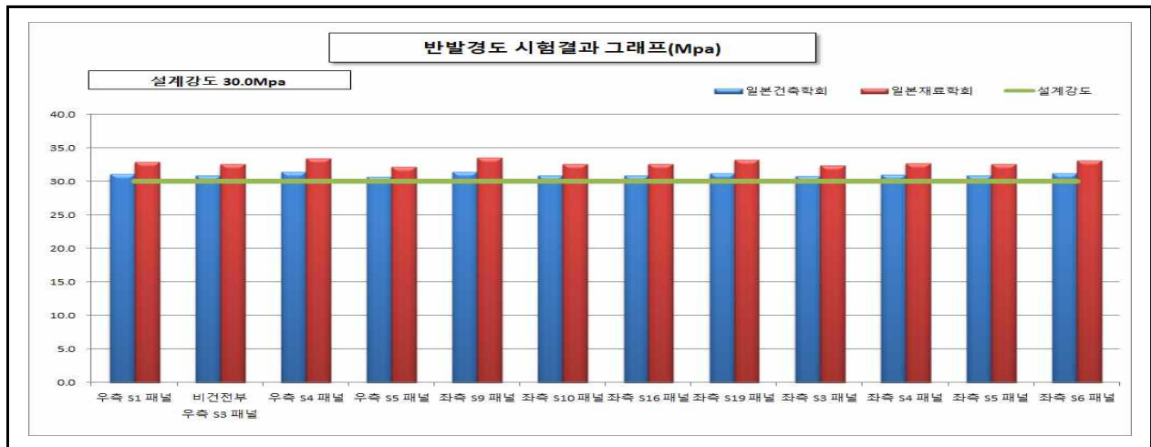
【그림 78.7】 반발경도시험 측정결과
