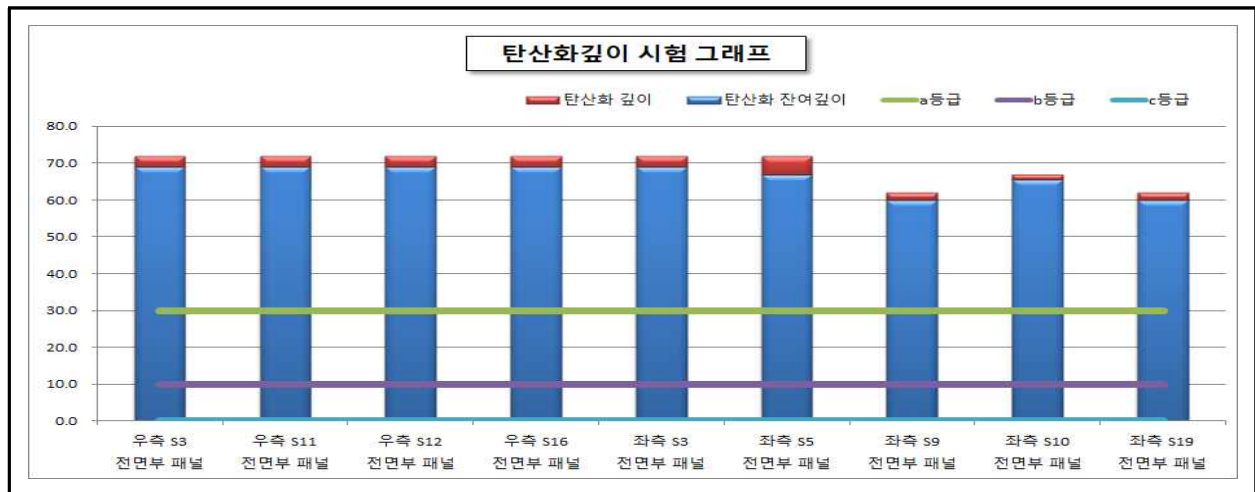
【그림 78.8】 탄산화 깊이 측정결과
