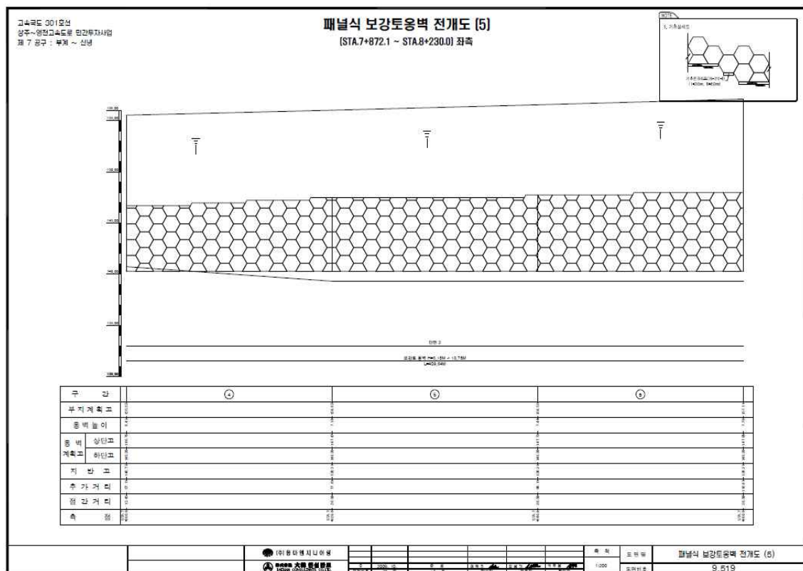
【그림 78.4】전개도
