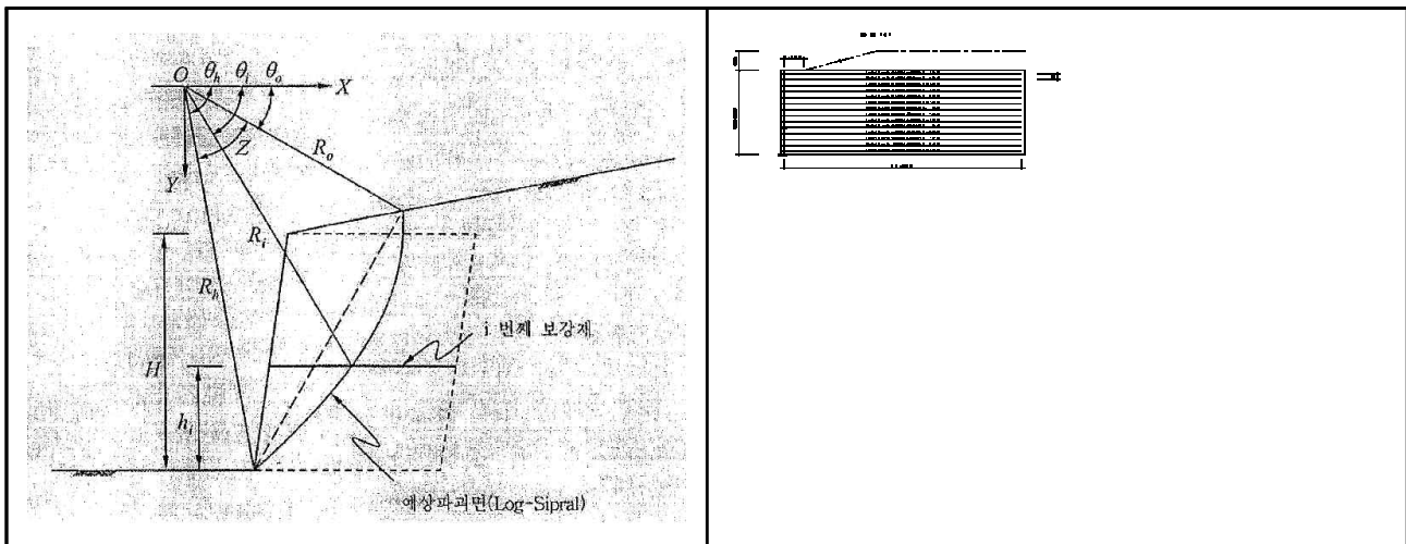
【그림 78.11】 토압작용 모식도
